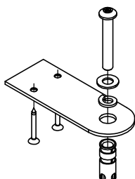
Ancrage antiivol en inox. SS antiitheft anchor. (Option # OANS-1PB04)
