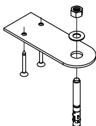
Ancrage std en inox. SS standard anchor. (Option # OANS-0PB04)
